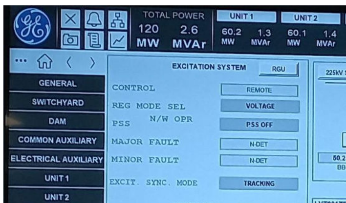
Vue partielle d'un des écrans de contrôle de l'IHM (Interface Homme Machine de l'automatisme)
