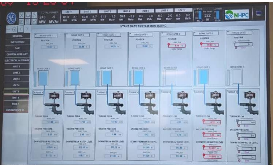
Photo de l'écran de contrôle de l'aménagement hydroélectrique de Nachtigal
